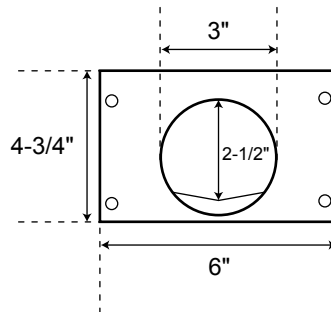
Outlet End
